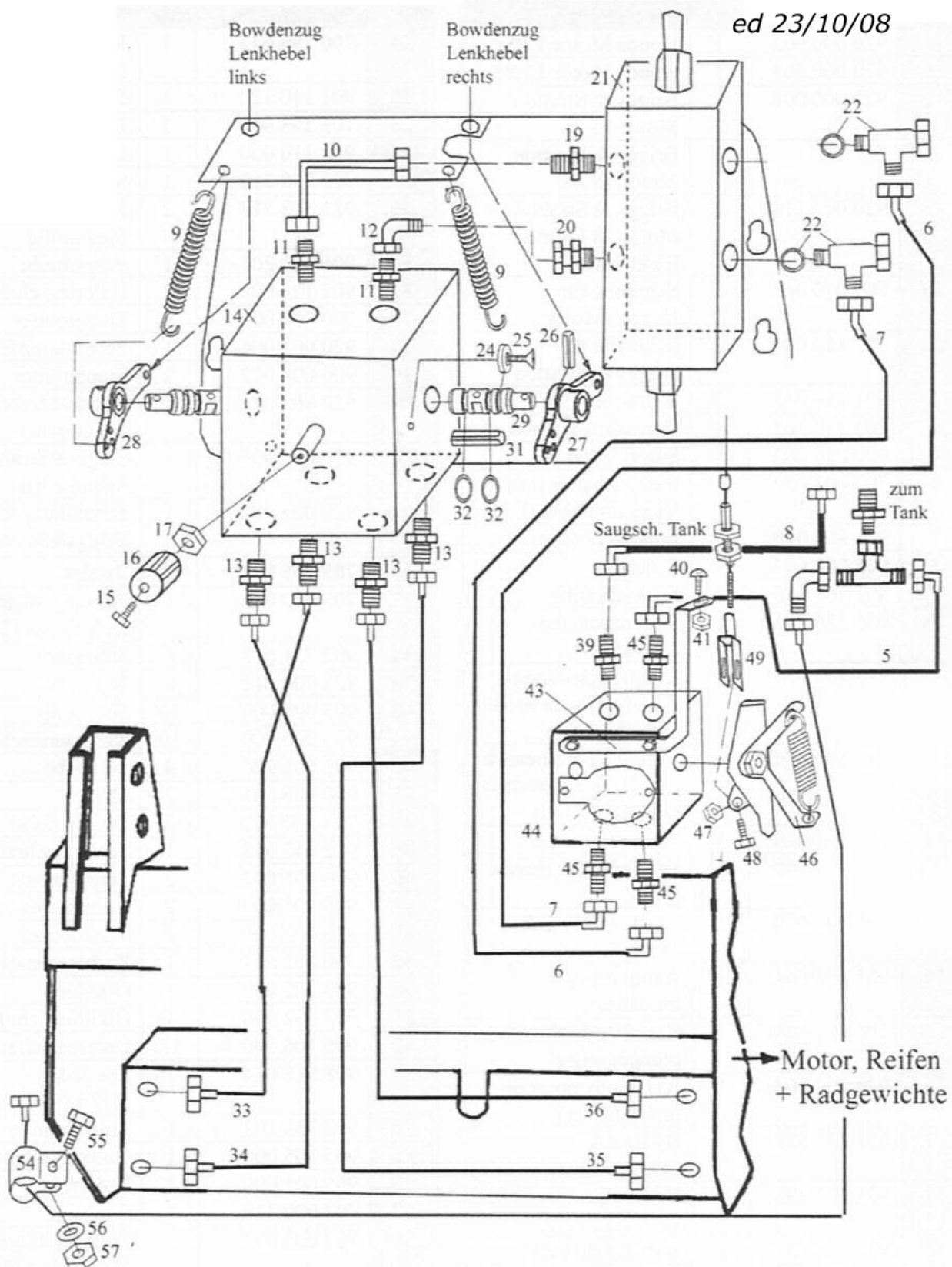
Eclaté 8 Circuit hydraulique après N° 36336 et après 39128 pour la conduite de drain
