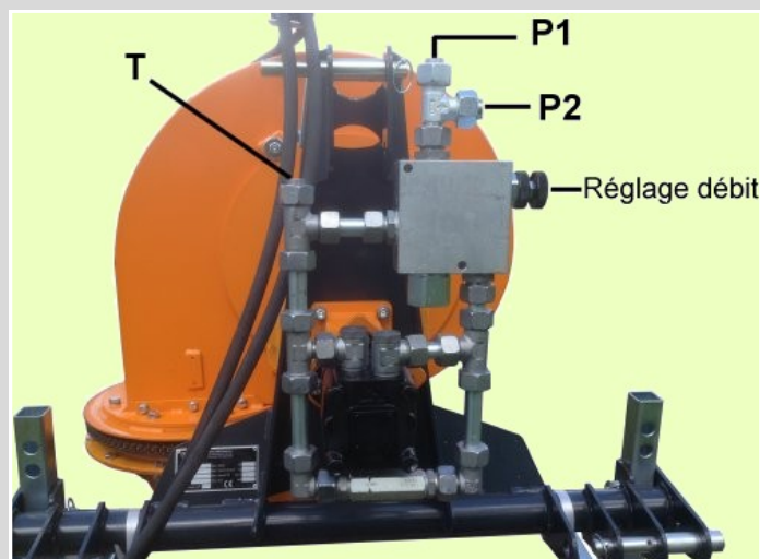
Raccordement hydraulique avec vanne de réglage de débit
